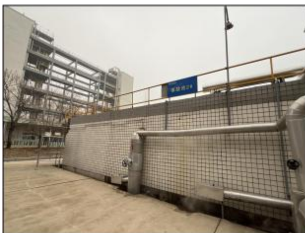
事故水池、雨污切换阀
